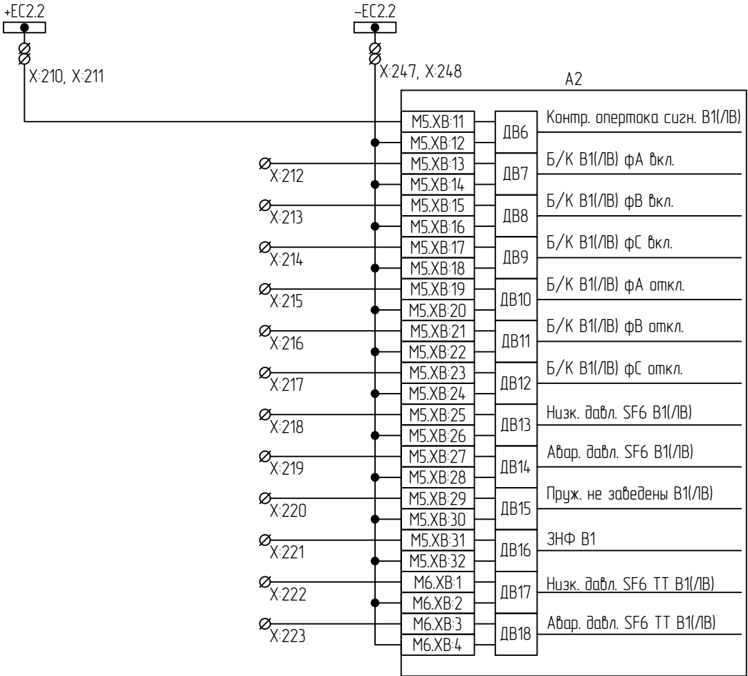
Цепи оперативного тока сигнализации выключателя и ТТ
