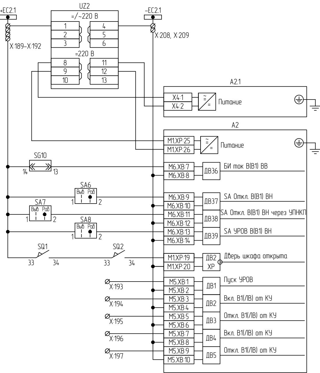
Цепи оперативного тока
